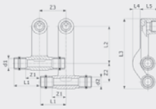
Соединительный элемент для подключения радиатора Sanpress - бронза Модель 2273.1
