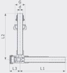
Соединительный комплект для подключения радиатора - латунь никелированная Модель 2272.5
